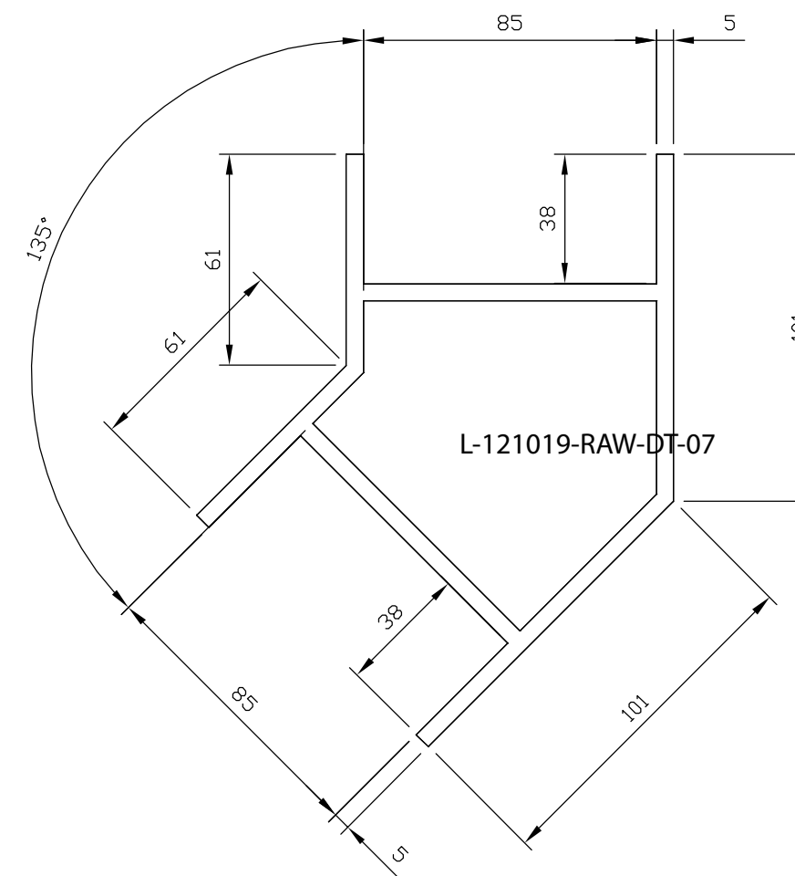
SECTION D'ANGLE 45° STANDARD L-121019-RAW-DT-05
