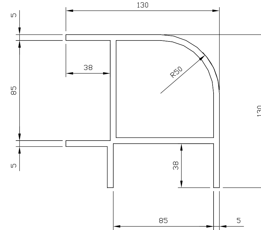
SECTION D'ANGLE 90° STANDARD L-121019-RAW-DT-06
