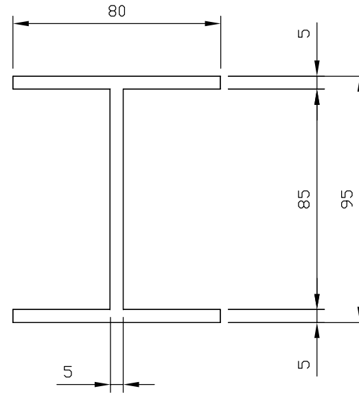
SECTION D'ASSEMBLAGE STANDARD L-121019-RAW-DT-07
